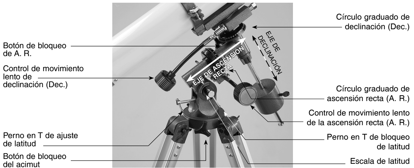
Figura 4. Montura ecuatorial.
