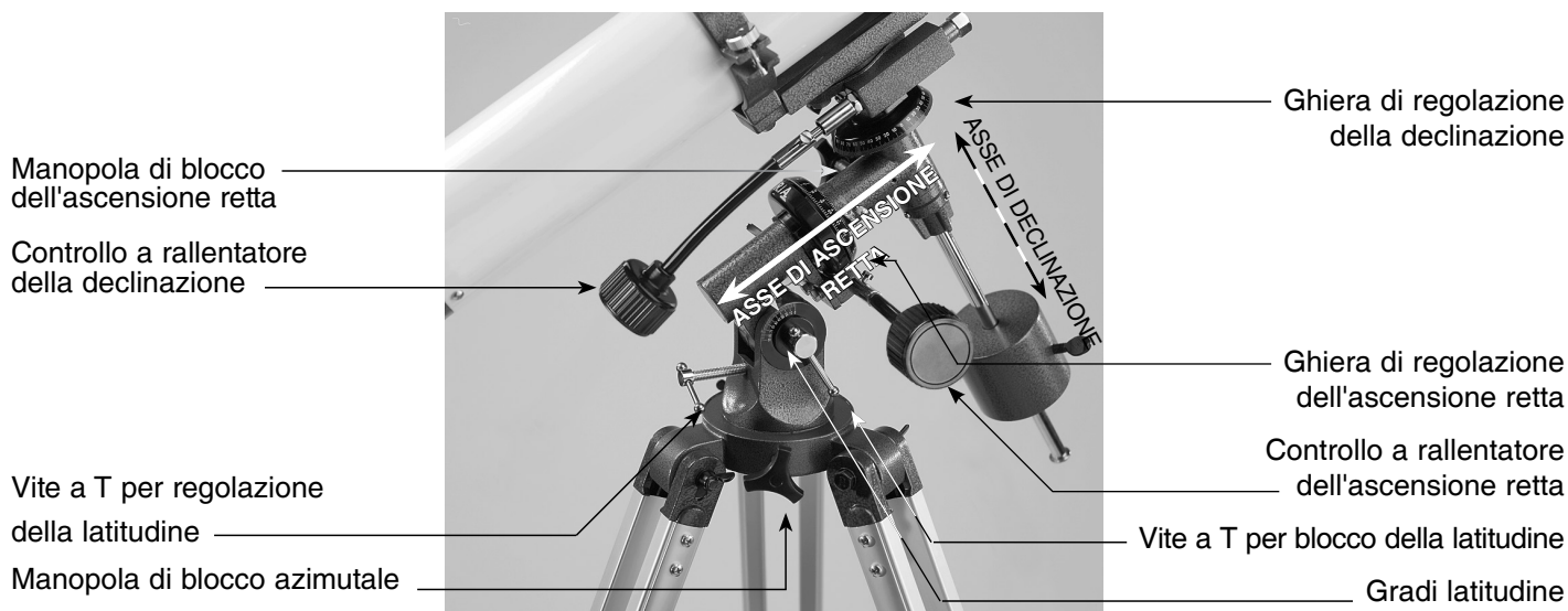
Figura 4. Montatura equatoriale.
