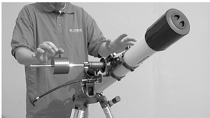
Figura 3b. Il telescopio ora è in equilibrio sull'asse dell'ascensione retta, ossia quando le mani lasciano la presa, la barra di contrappeso rimane orizzontale.
