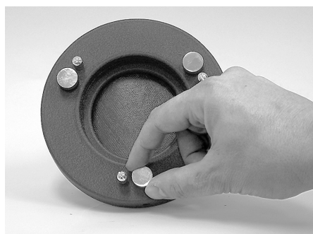
Abbildung 15. Die Neigung des Primärspiegels wird durch Drehen der drei größeren Rändelschrauben eingestellt.
