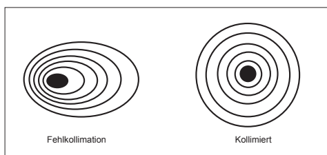
Abbildung 16. Mit einem Sternentest wird ermittelt, ob die Teleskopoptik richtig kollimiert ist. Wenn die Optik perfekt kollimiert ist, sollte eine
