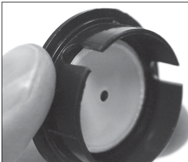
Abbildung 12. Die Schnellkollimationskappe, die über eine reflektierende Innenfläche verfügt, hilft während der Kollimation beim Zentrieren der Reflexionen der Optik zum Fokussierer.
